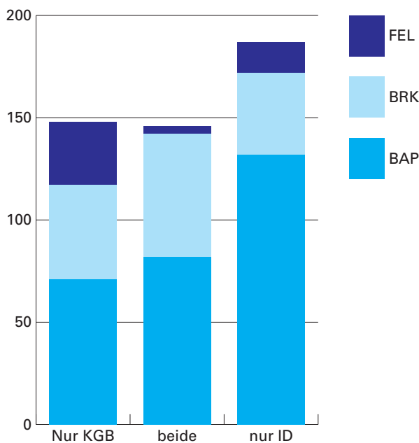
Abb. 10: Anzahl Kilometerquadrate (Nord- und Mittelbündens zwischen 1200 und 2100 m ü.M.) aus denen in den Jahren 2000 bis 2013 Bruthinweise der drei Fokusarten gemeldet wurden. Cyan: Quadrate, aus welchen Nachweise nur im Rahmen der vorliegenden Untersuchung gelangen; hellblau: Quadrate, aus denen zusätzlich Nachweise in der ID-Datenbank vorhanden sind; Dunkelblau: Quadrate, die im Rahmen der vorliegenden Untersuchung nicht besucht wurden, aus denen aber Bruthinweise der entsprechenden Fokusart eingingen. Zu beachten ist, dass Bruthinweise von Baumpieper und Braunkehlchen durch die freiwilligen Mitarbeiter der Vogelwarte gemeldet werden müssen, während dies bei der Feldlerche freiwillig ist. Der dunkelblaue Abschnitt der Feldlerchensäule wäre bei gleichen Vorschriften für alle drei Arten deshalb vermutlich höher.
